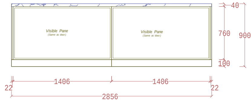
ELEVATION B
